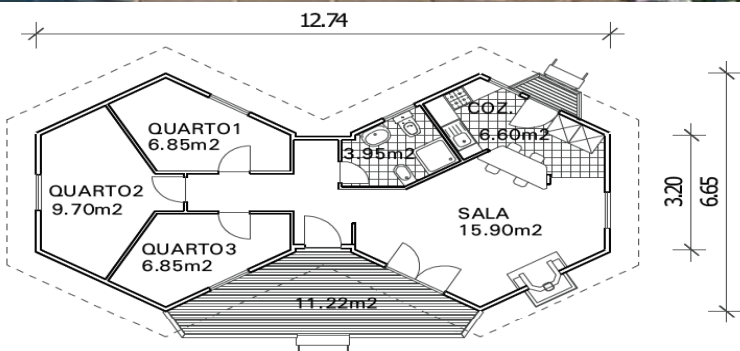
PLANTA T3 65 65.00 m2
